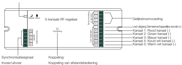
Aansluitmodule master/slave
