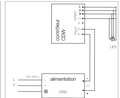
câblage CDW
